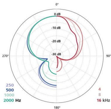
MiniCMIT ポーラーパターン
