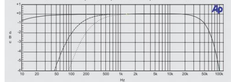
50 kHz まで -1dB をキープするフラット特性。
